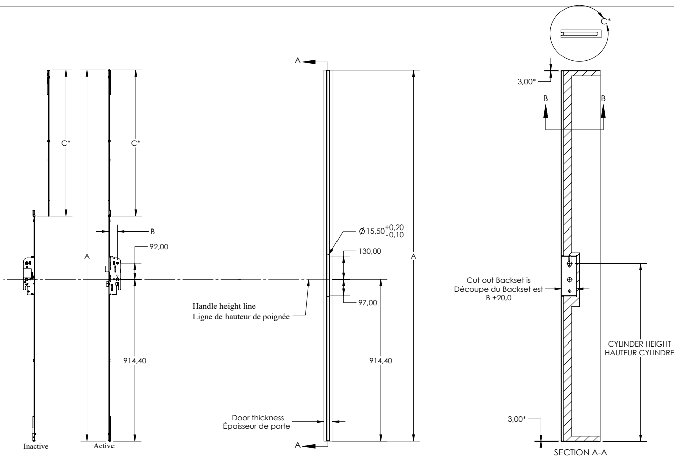
ACTIVE & INACTIVE DOOR PANELS / PANNEAUX DE PORTE ACTIF ET INACTIF
